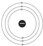
میدان مغناطیسی
