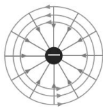
میدان الکترومغناطیس
